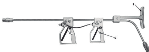
Pistola de aplicación con capacidad de operar en un rango de hasta 40.000 psi
